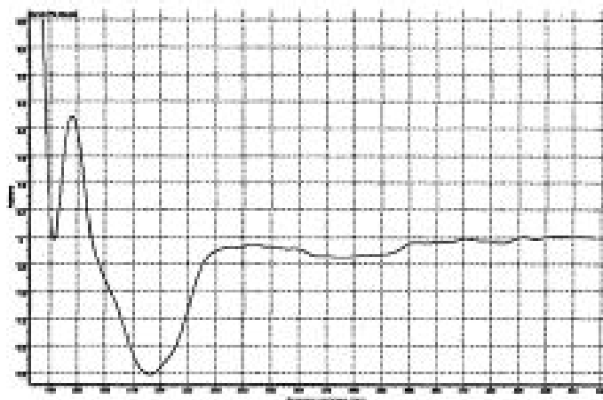
Слика 1: CD спектар на (R)-4-[4-бромофенил]-2,2-диметил-1,3-диоксолан
